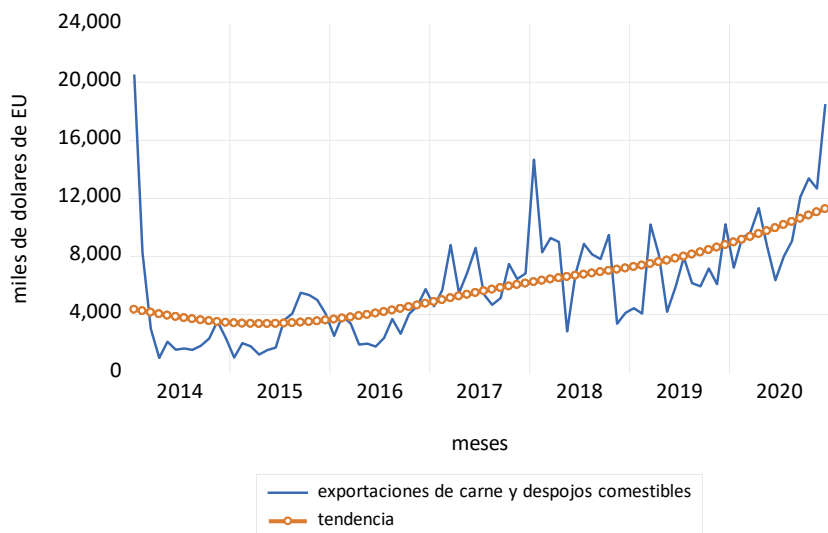
Gráfica 2. Colombia. Tendencia de las exportaciones de carne y despojos comestibles según el filtro de Hodrick-Prescott, enero/2014-dicbre/2020
