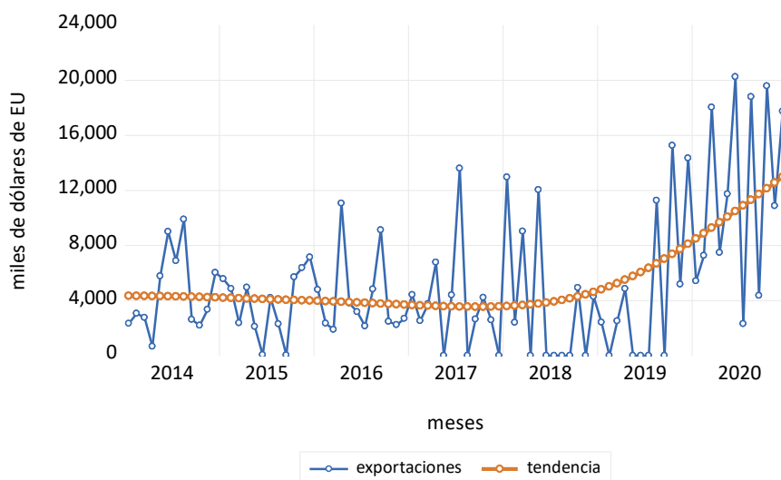
Gráfica 1. Colombia. Tendencia de las exportaciones de ganado vacuno vivo según el filtro de Hodrick-Prescott, enero/2014-dicbre/2020.
