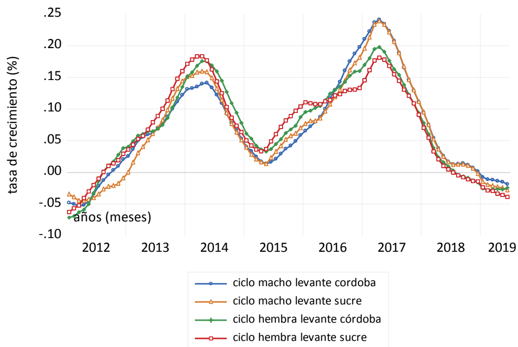
Gráfica 1. Córdoba-Sucre. Ciclo del precio del ganado de levante macho y hembra enero/2012 a junio/2019
