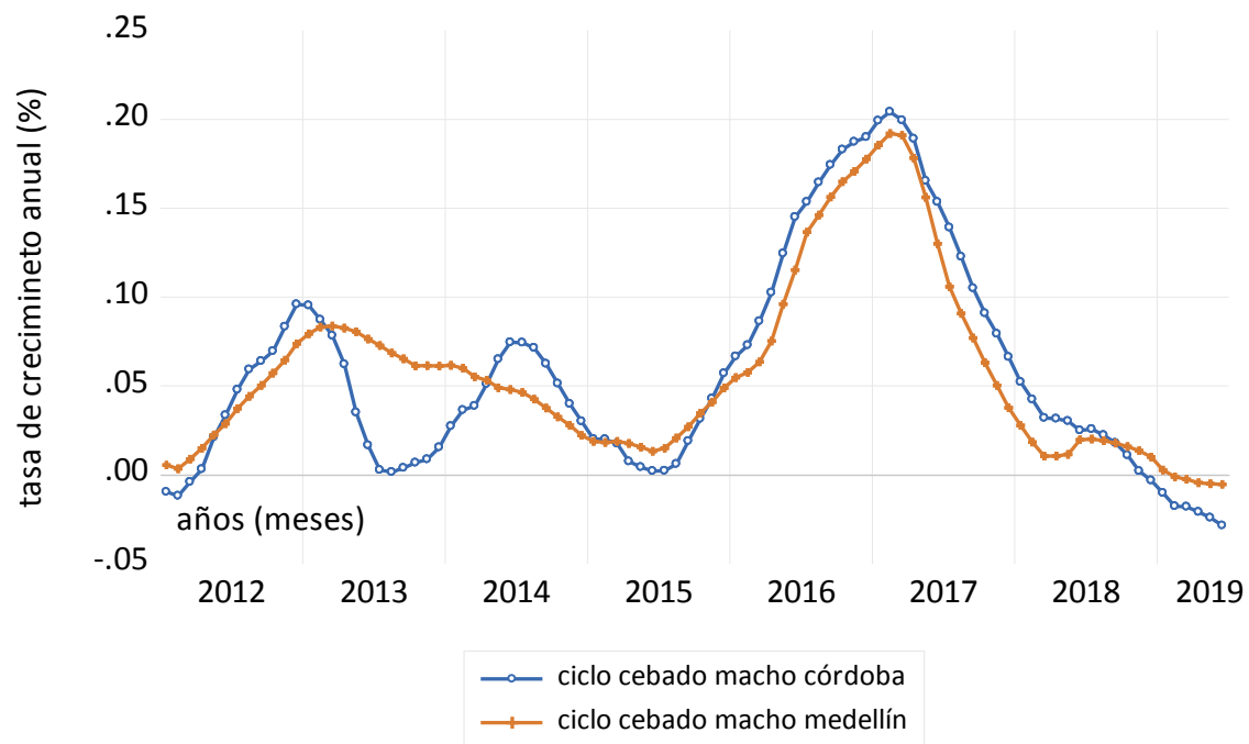
Gráfica 2. Córdoba-Medellín. Ciclo del precio del ganado vacuno vivo cebado, enero/2012 a junio/2019
